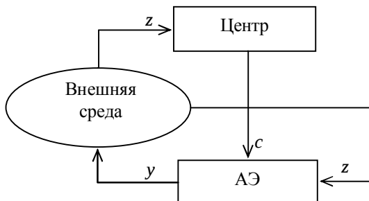
Рис. 3.1. Модель активной системы с внешней неопределенностью и симметричной информированностью
