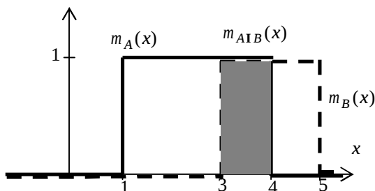
Рис. 4.3. Пересечение множеств
