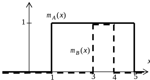
Рис. 4.2. Включение нечетких множеств
