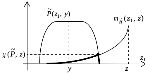
Рис. 4.7. Эскизы функций принадлежности информационного множества \tilde{P} , отношения предпочтения \tilde{R} и значения g(\tilde{P}, z) .
