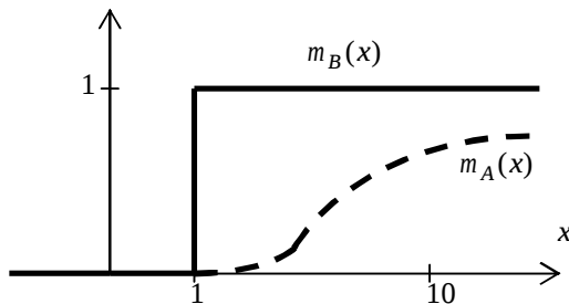
Рис. 4.1. Пример четкого
