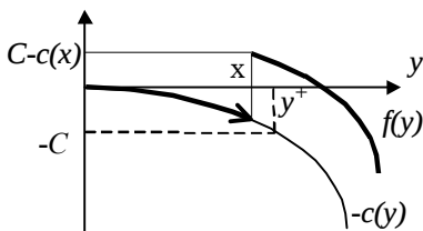
Рис. 2.6. Целевая функция АЭ при использовании центром системы стимулирования С-типа
