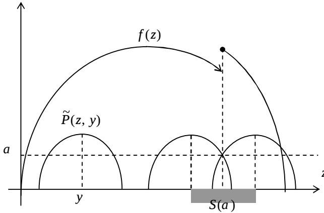
Рис. 4.8. Функция полезности АЭ в задаче стимулирования с нечеткой неопределенностью.
