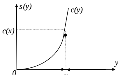
Рис.2.3. Квазискачкообразная система стимулирования
