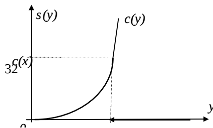
Рис. 2.2. Скачкообразная система стимулирования
