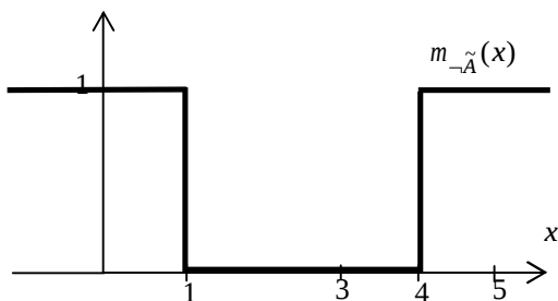
Рис. 4.5. Дополнение множества
