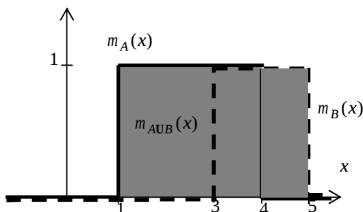
Рис. 4.4. Объединение множеств
