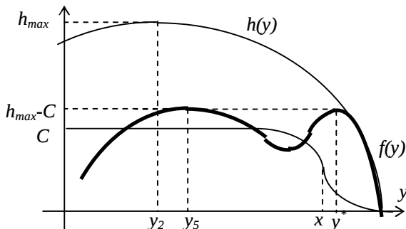
Рис. 3.2. Целевая функция A\hat{E} в задаче теории контрактов
