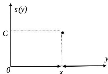
Рис.2.3. Квазискачкообразная система стимулирования
