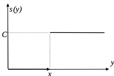
Рис. 2.2. Скачкообразная система стимулирования
